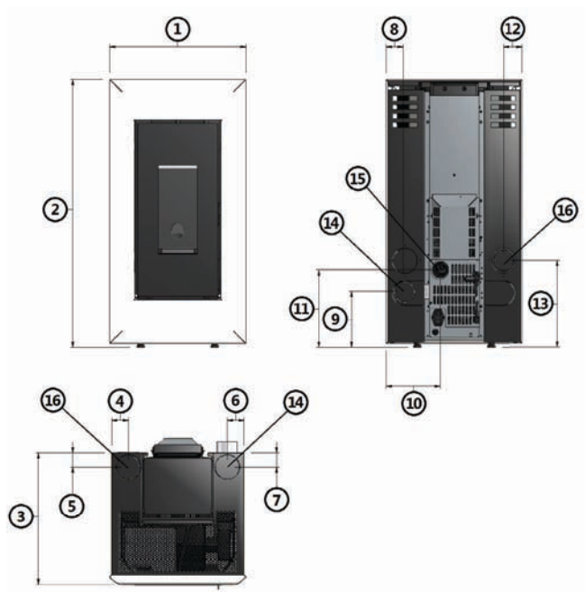
Fig. 17 - Dimensions générales: Vega / Trend
