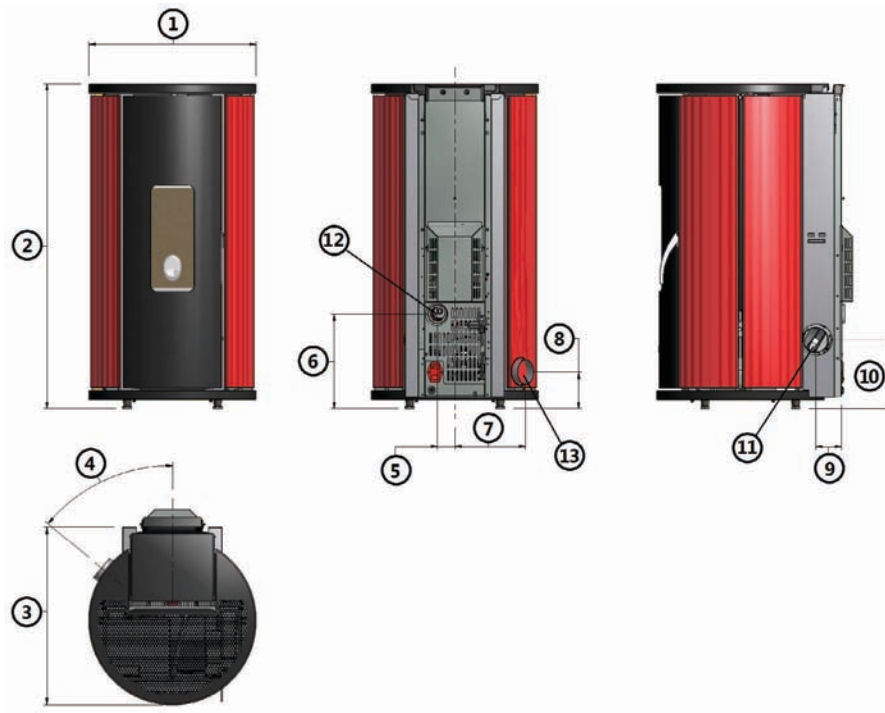
Fig. 20 - Dimensions générales: Sfera³ / Sfera³ Plus / Globe
