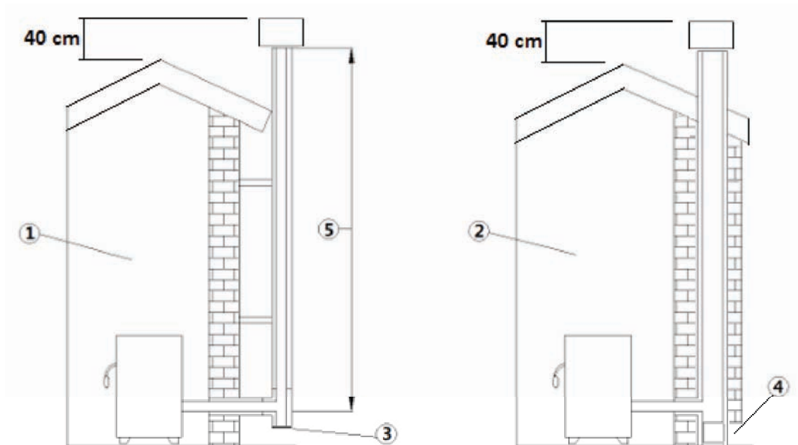
Fig. 1 - Conduit des fumées
