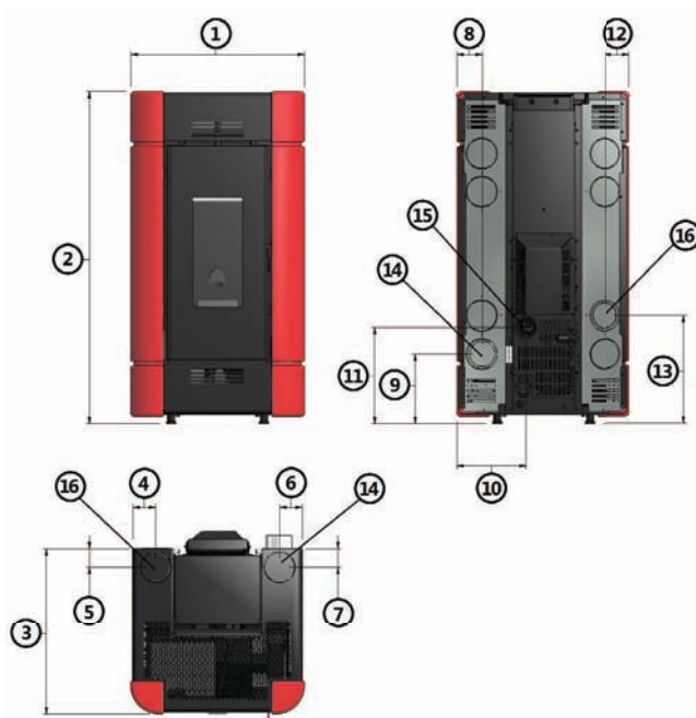
Fig. 18 - Dimensions générales: Sire³ Plus
