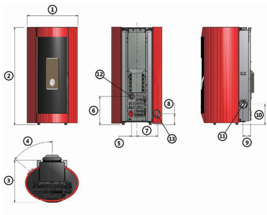
Fig. 22 - Dimensions générales: Elise 3 Plus
