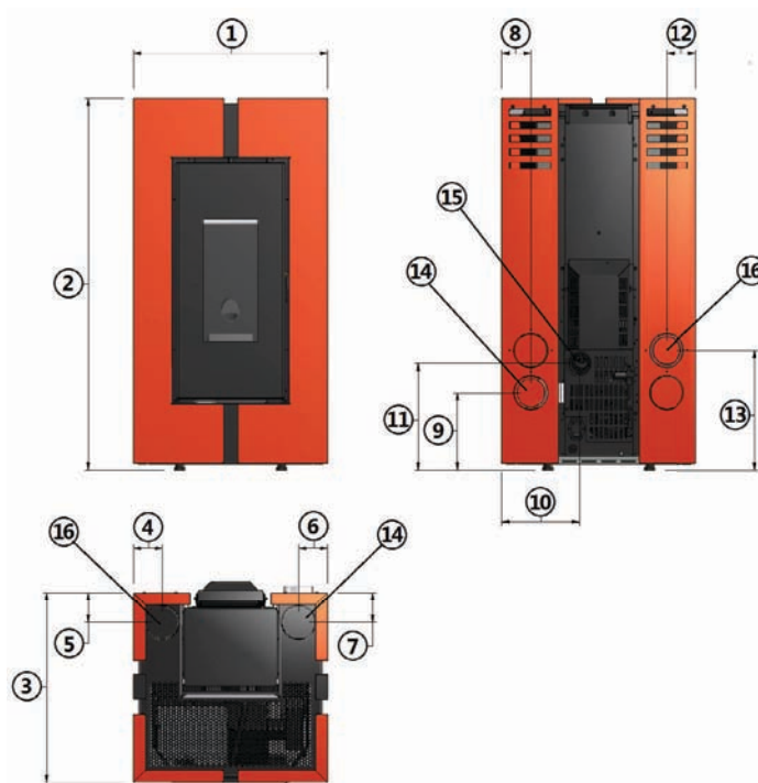
Fig. 19 - Dimensions générales: Doge³ Plus
