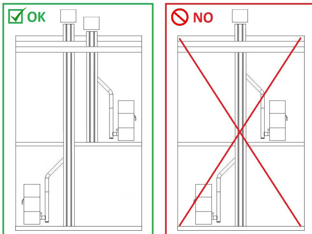
Fig. 16 - Exemples des installation correcte
