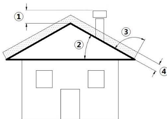
Fig. 2 - Toit en pente
