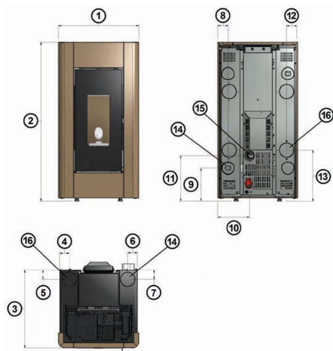
Fig. 21 - Dimensions générales: Prince³ / Prince³ Plus
