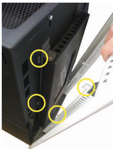
Fig. 24 - Assembler le panneau frontal
