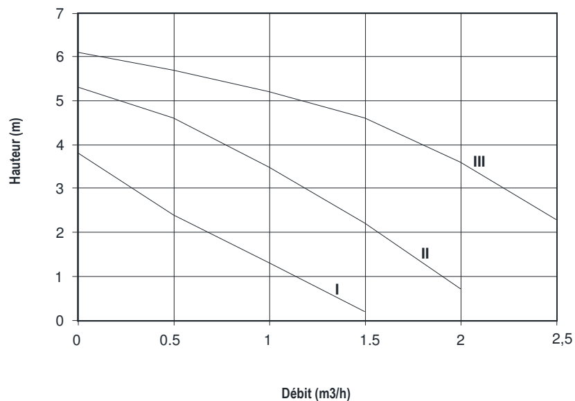
CIRCULATEUR DE RELANCE - Wilo RS 15/6 Ku
