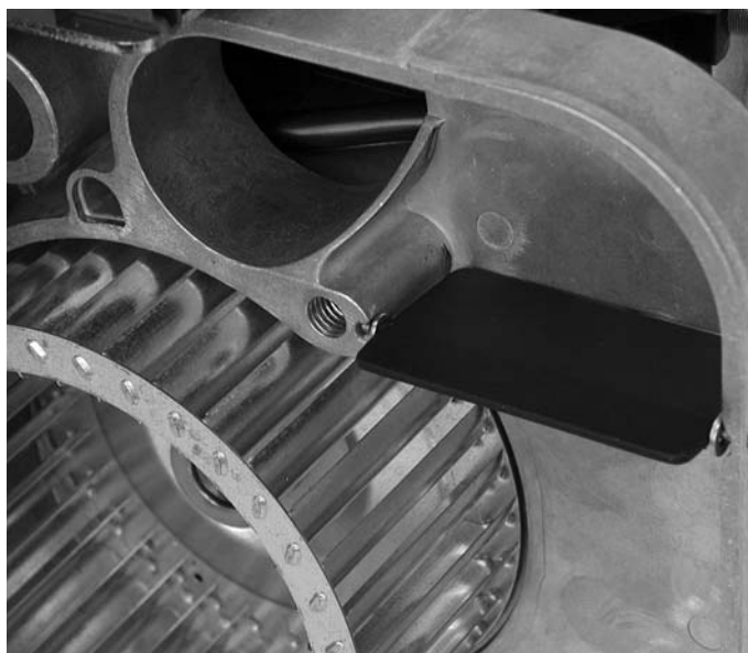
Figure 21 - Position de montage du clapet d'air
